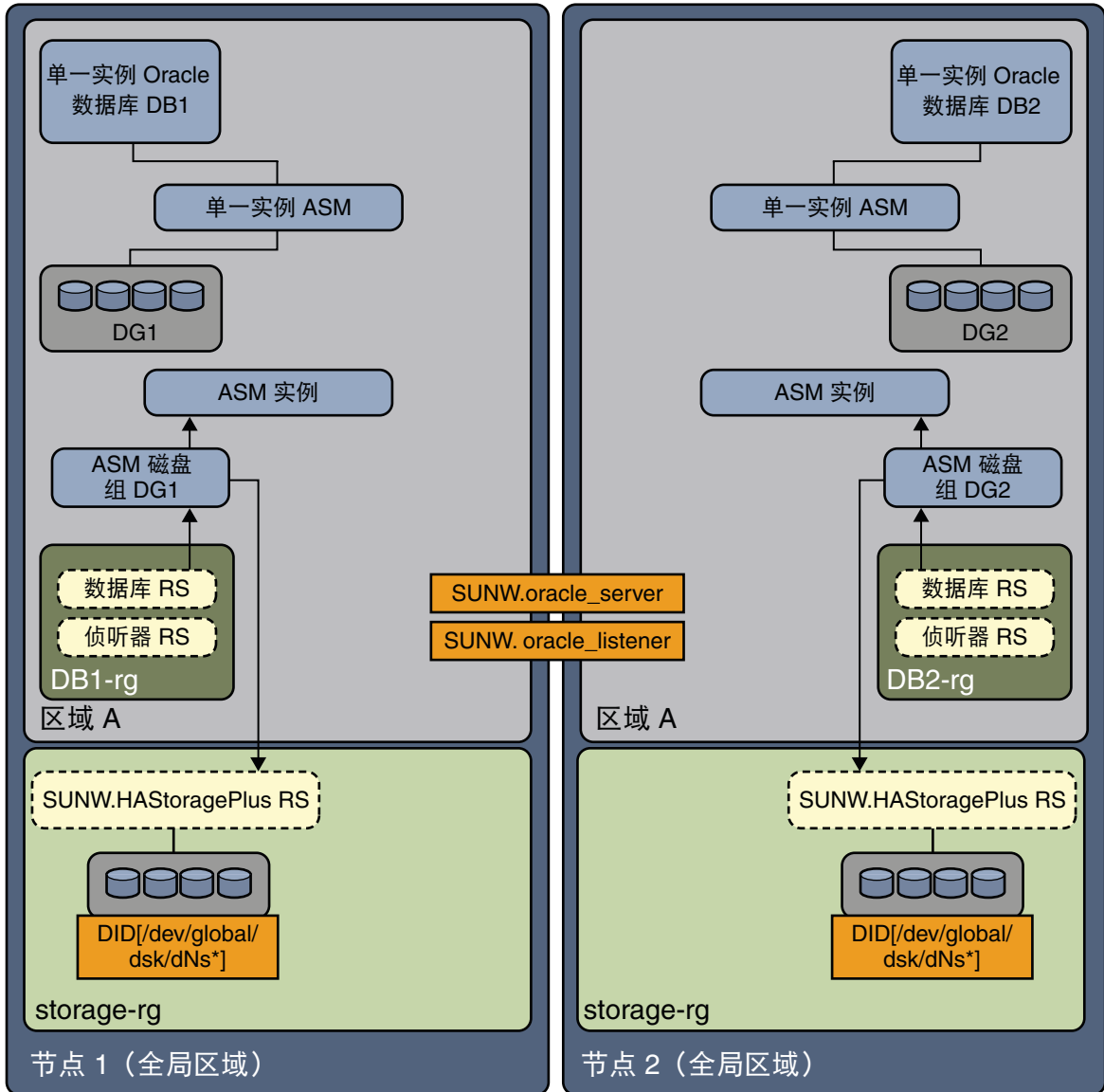
图 C-7 非全局区域中使用单独磁盘组的单实例 Oracle ASM [2]
