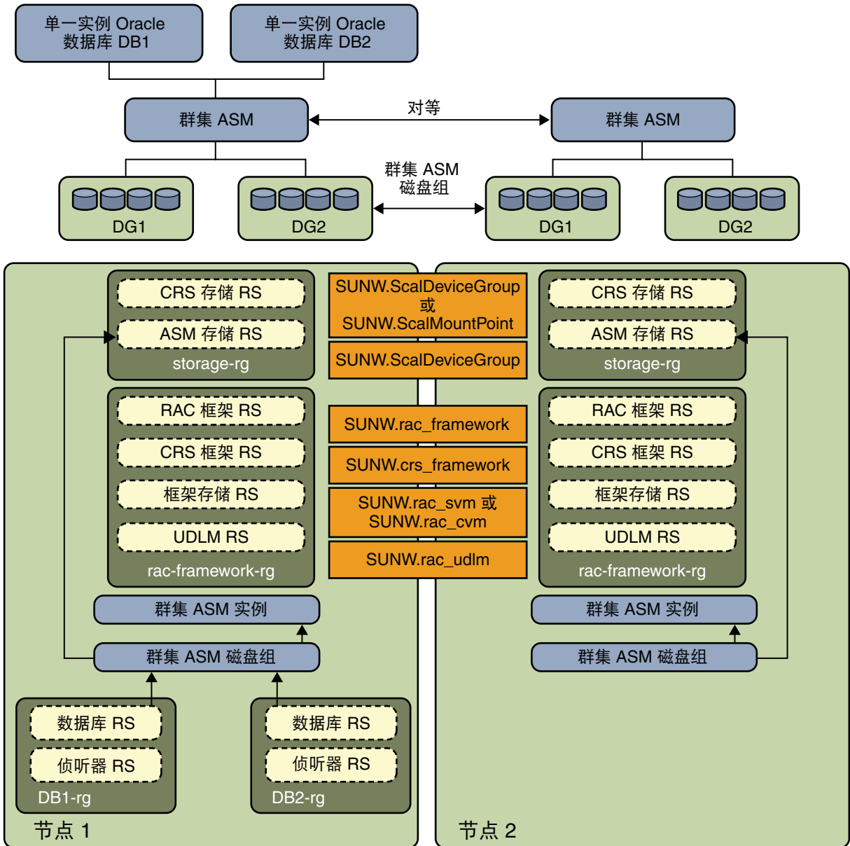
图 C-4 使用群集磁盘组的群集 Oracle ASM [1]
