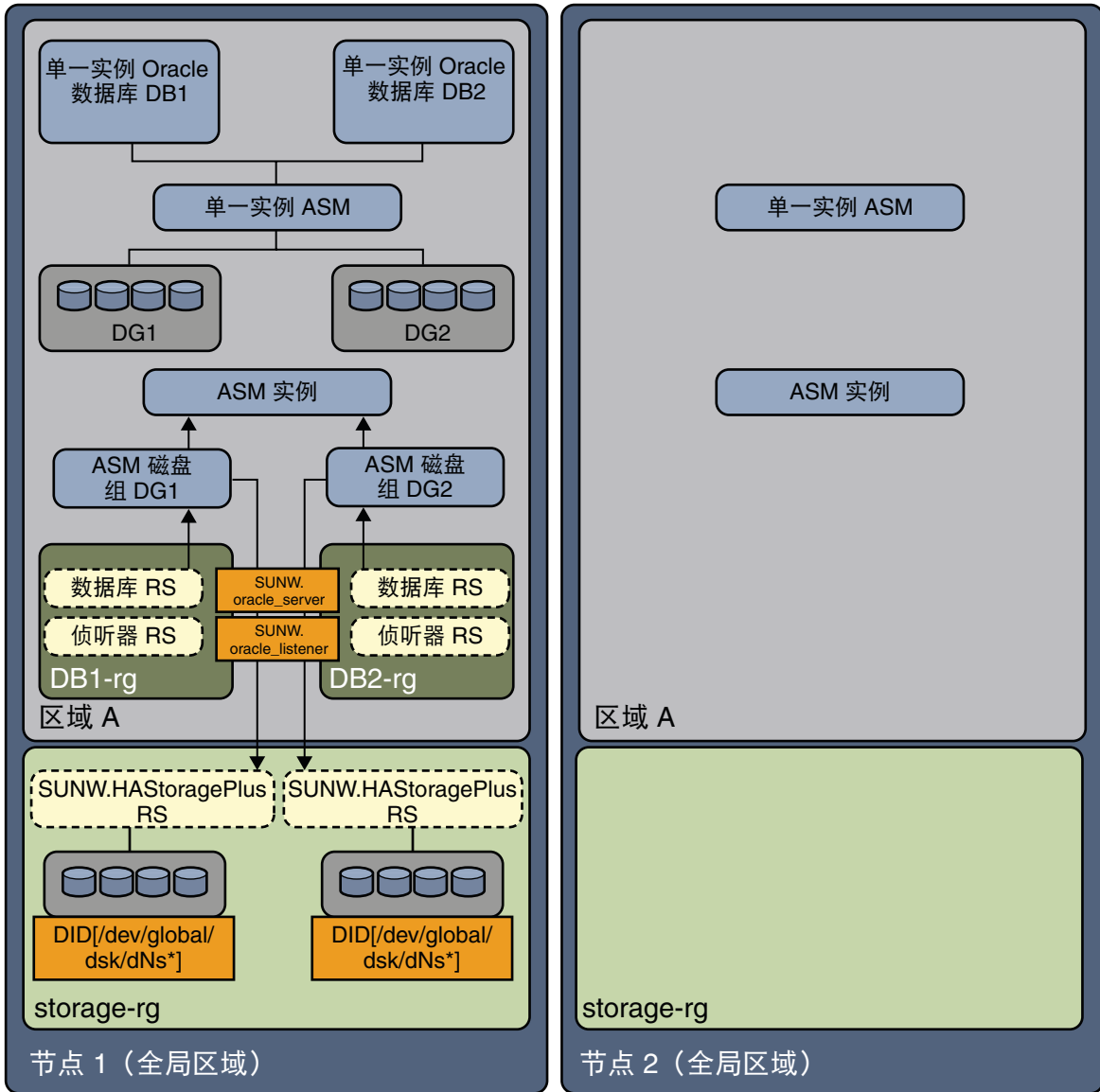
图 C-6 非全局区域中使用单独磁盘组的单实例 Oracle ASM [1]
