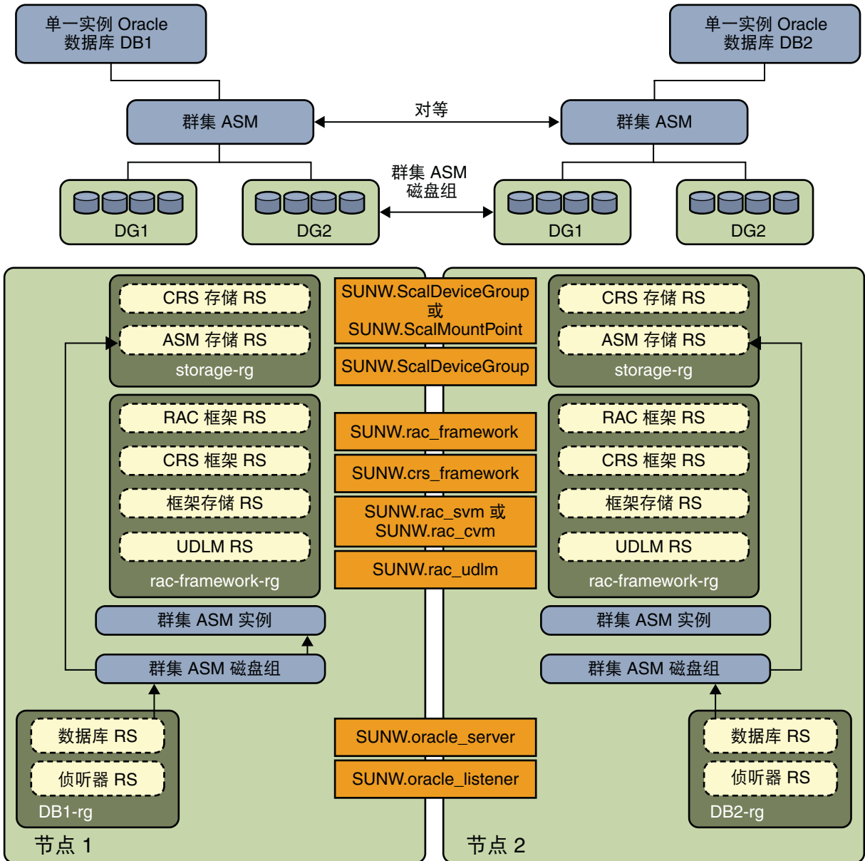
图 C-5 使用群集磁盘组的群集 Oracle ASM [2]
