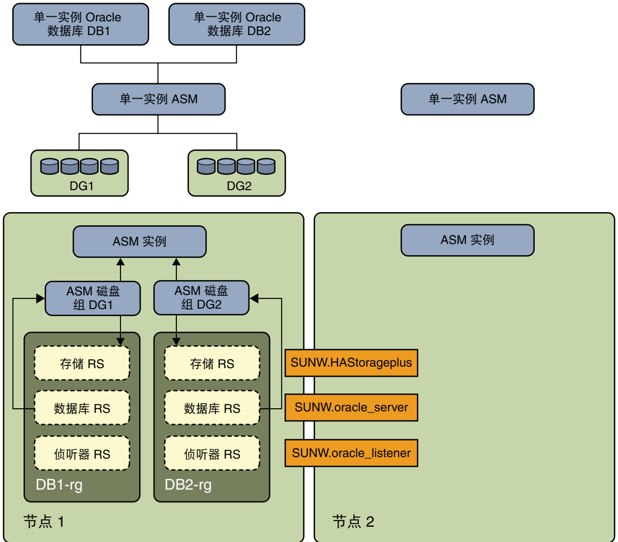
图 C-2 使用单独磁盘组的单实例 Oracle ASM [1]
